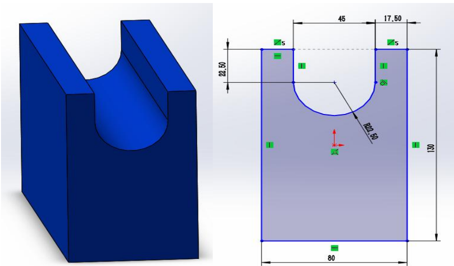
图8 管道槽
